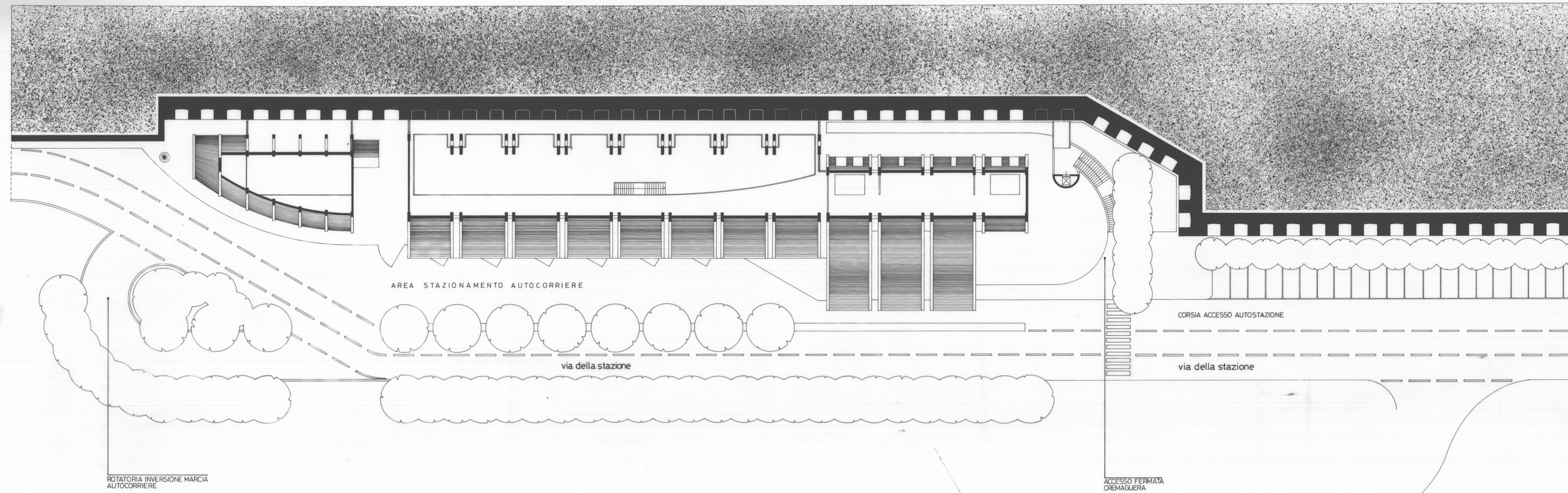
PIANTA QUOTA SOPPALCHI scala 1:200
